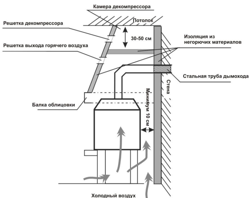
РИСУНОК 4: ВИД СБОКУ
